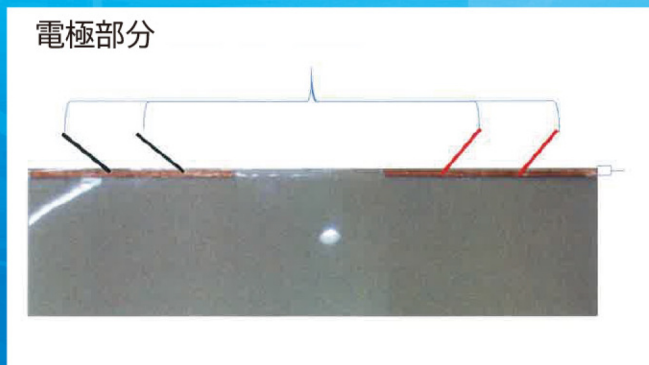
電極部分 一枚のフィルムに対して、左右2箇所 に電極が取り付けられておりそれぞれの 電極に配線が2本ずつ結線されている
